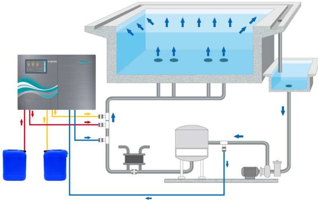
Anschluss-Schema für den PoolManager®
